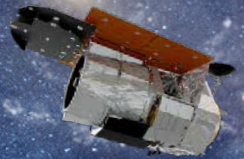
Roman 2025/2026
