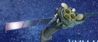
XMM-Newton (ESA) 12/10/1999
