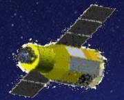
XRISM (JAXA) 2022
