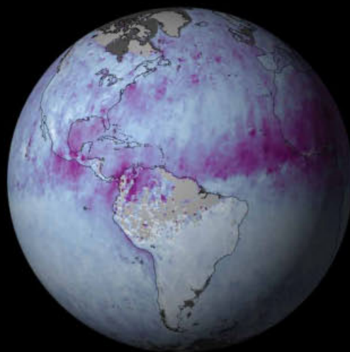
MISR Aerosols
